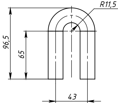
Поз.3 (Ушко)
